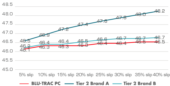
Longitudinal Aquaplaning
